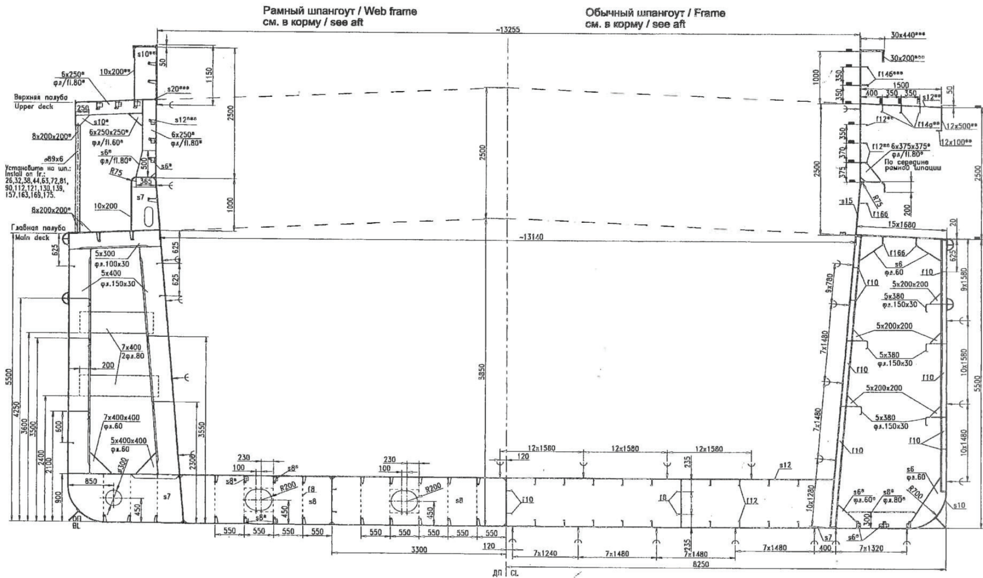
Рисунок 1.2. Схема поперечного сечения трюмов. Figure 1.2. Transverse section of cargo holds.
